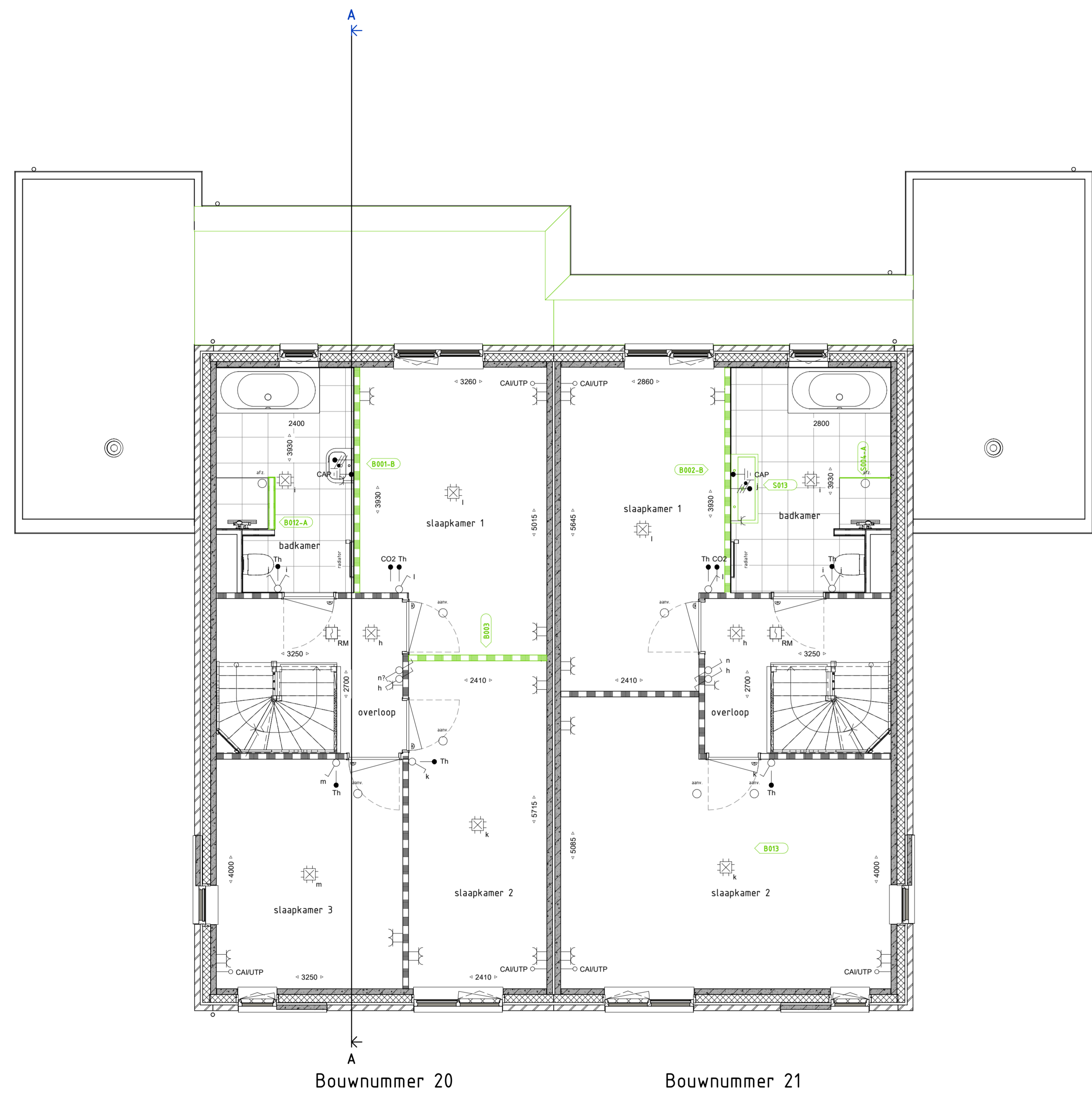
EERSTE VERDIEPING 1 : 50
