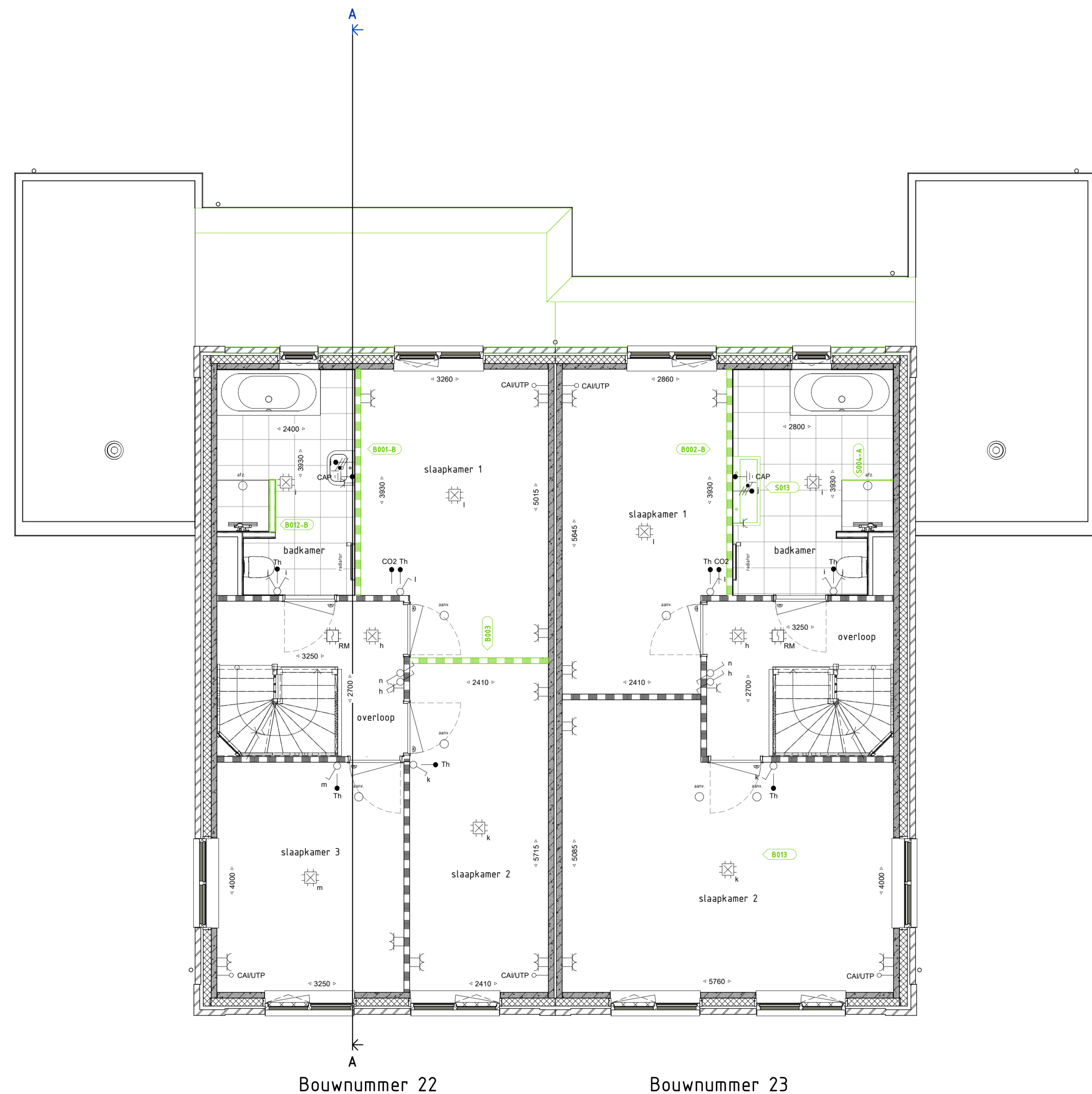
EERSTE VERDIEPING 1 : 50
