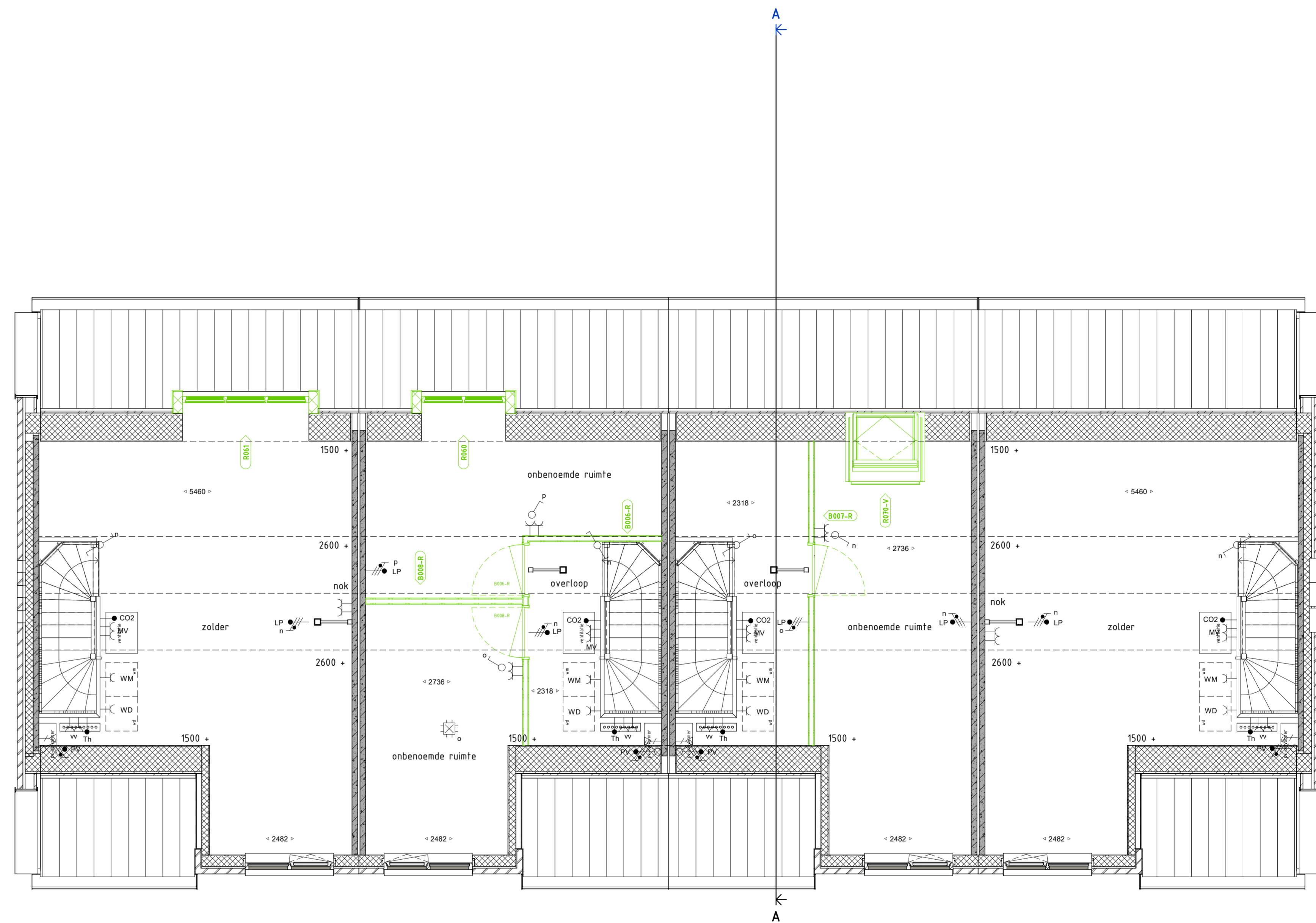
TWEDE VERDIEPING 1 : 50 Bouwnummer 27 Bouwnummer 28 Bouwnummer 29 Bouwnummer 30
