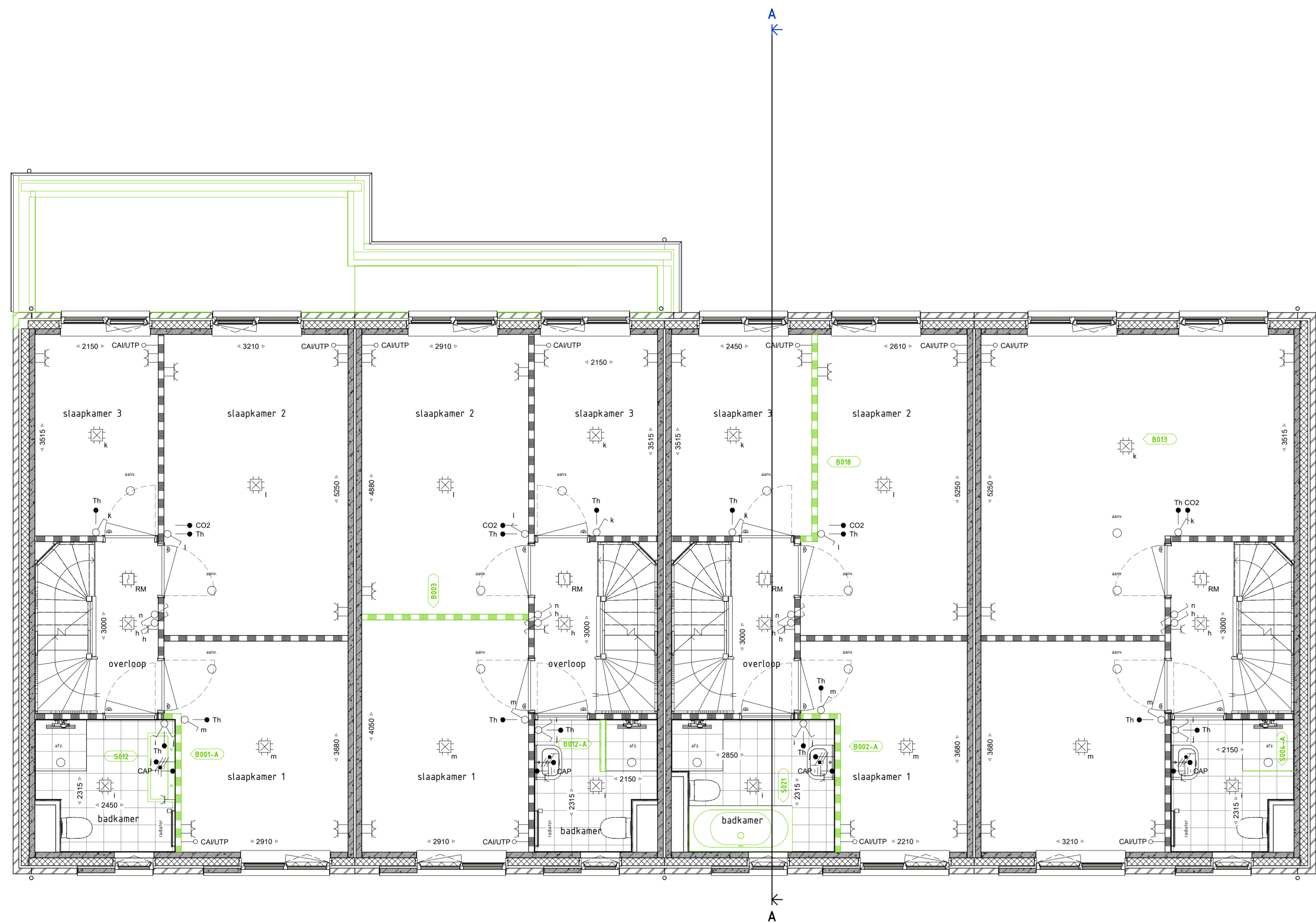
EERSTE VERDIEPING 1 : 50 Bouwnummer 27 Bouwnummer 28 Bouwnummer 29 Bouwnummer 30
