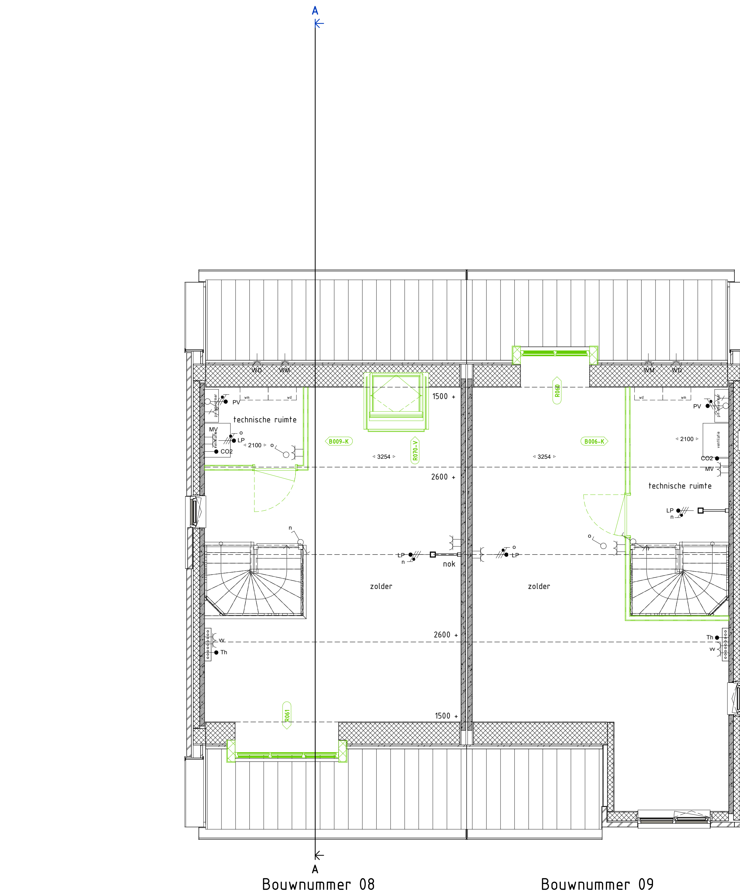
TWEDE VERDIEPING 1 : 50
