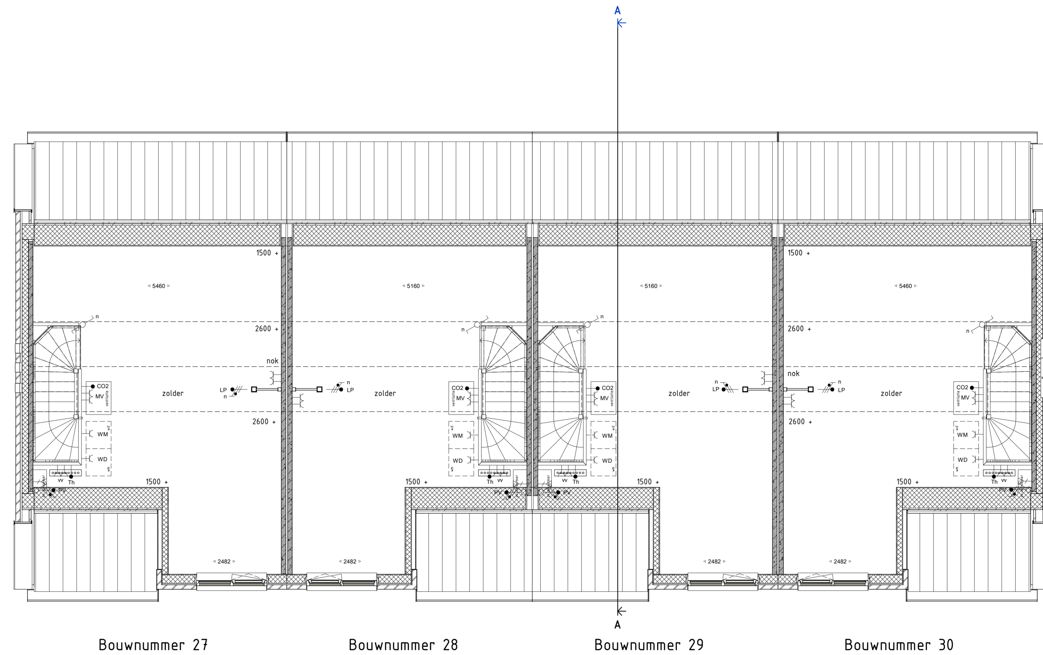
TWEDE VERDIEPING 1 : 50
