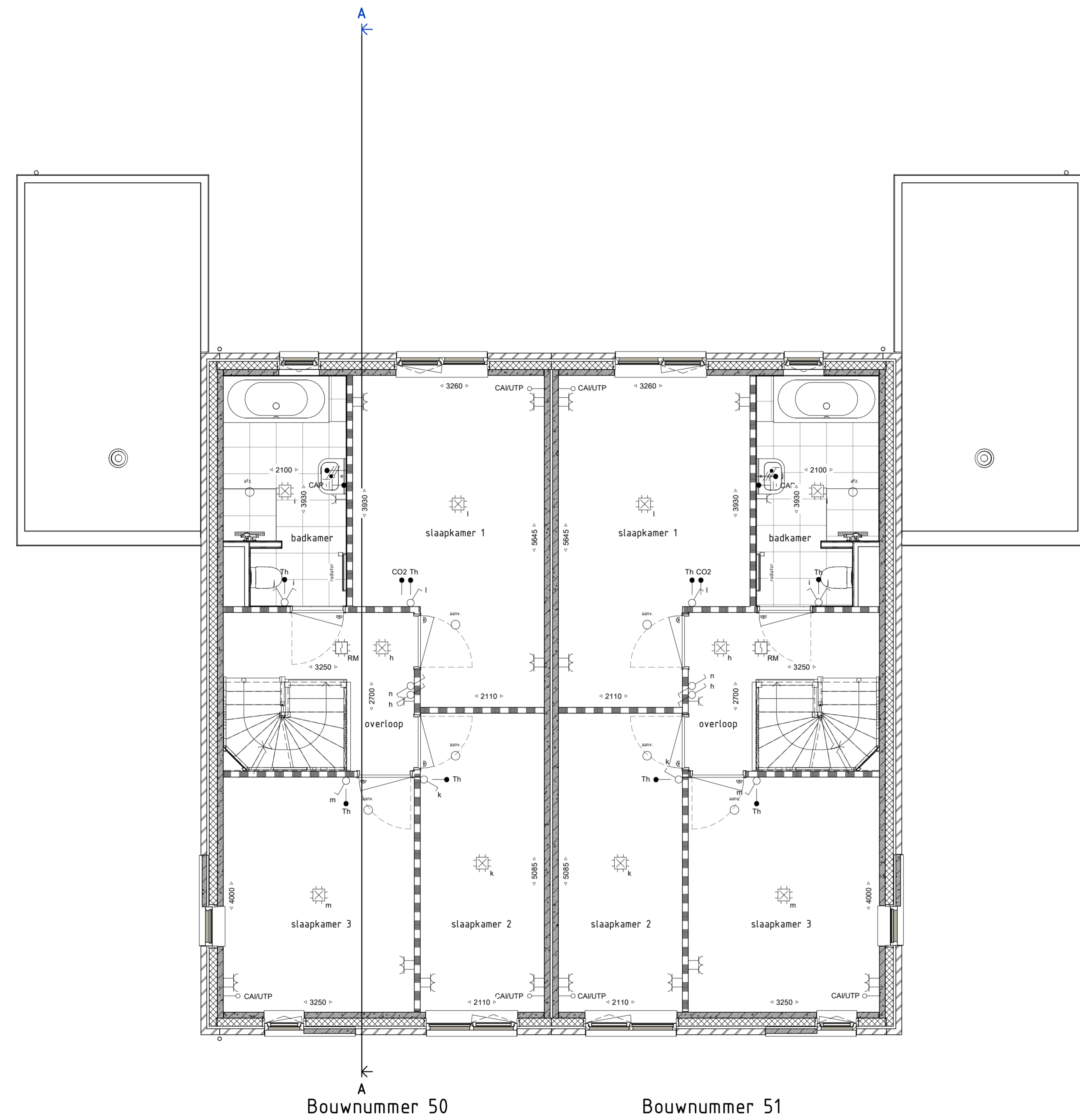
EERSTE VERDIEPING 1 : 50
