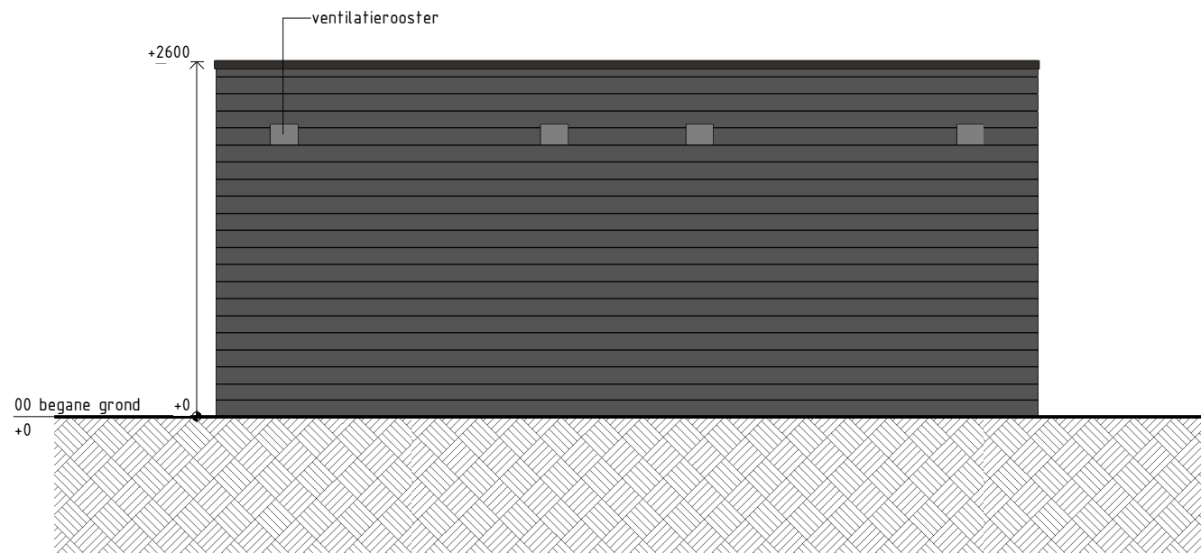
VOORGEVEL 1 : 50
