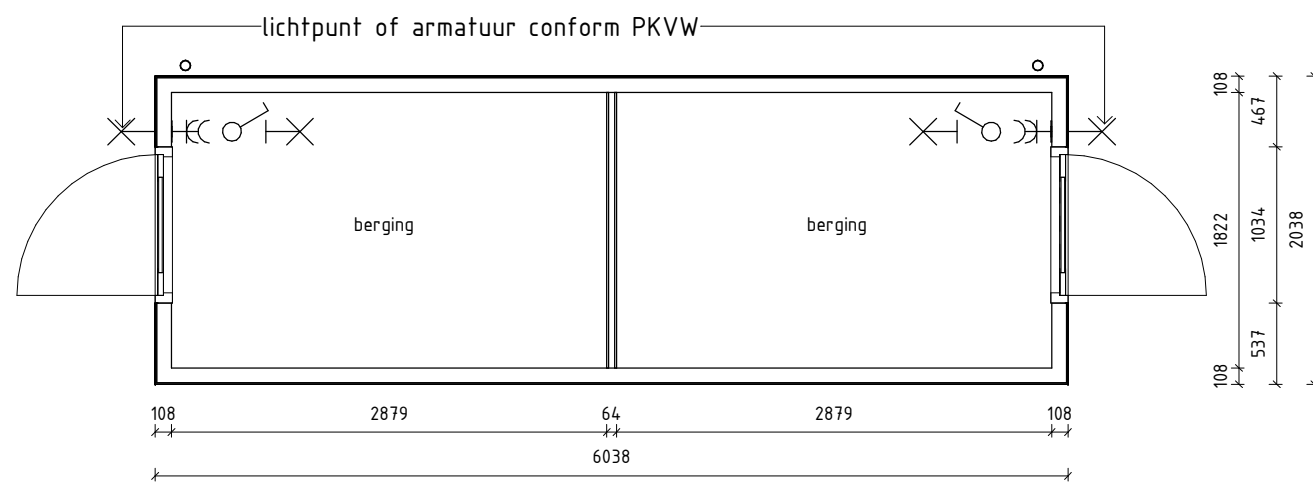
PLATTEGROND 1 : 50
