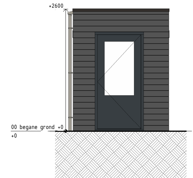
LINKERZIJGEVEL 1 : 50
