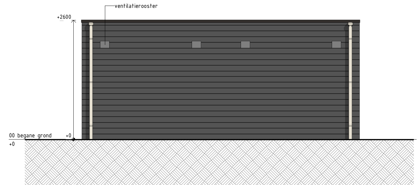
ACHTERGEVEL 1 : 50
