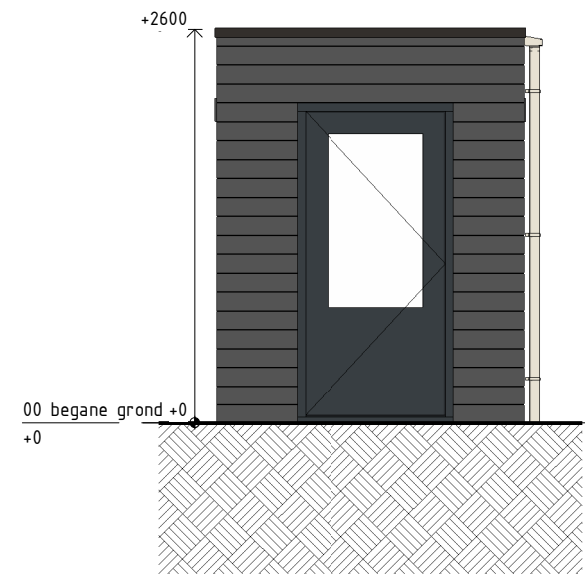
RECHTERZIJGEVEL 1 : 50
