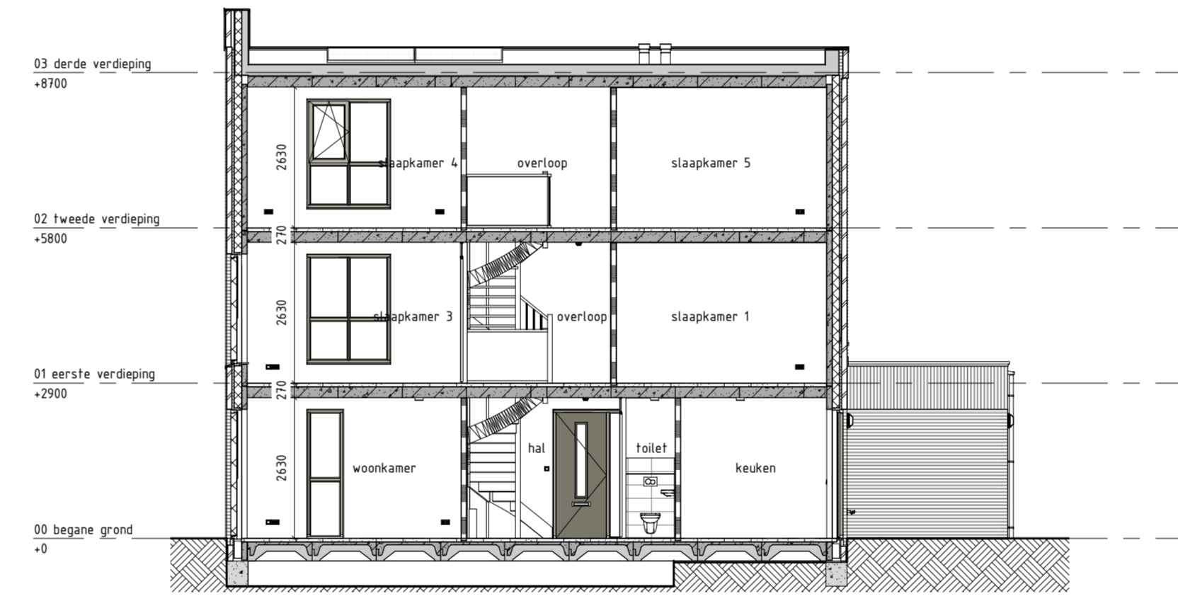
DOORSNEDE A 1 : 100
